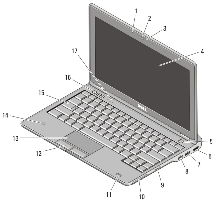
Figur 1. Set forfra
