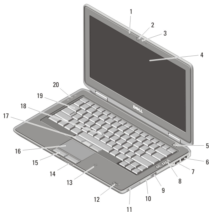
Figur 3. Set forfra
